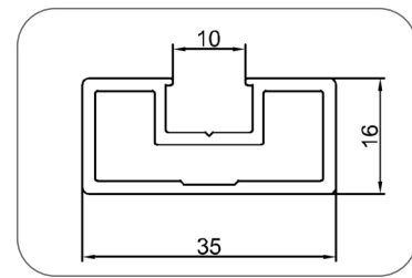
CASP-SP-3516 - DOOR FRAMED PROFILE
